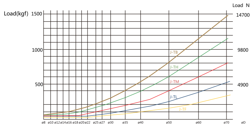
Numbers of bend: 1 million bend 100万次
